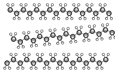
Poly(ethene)
